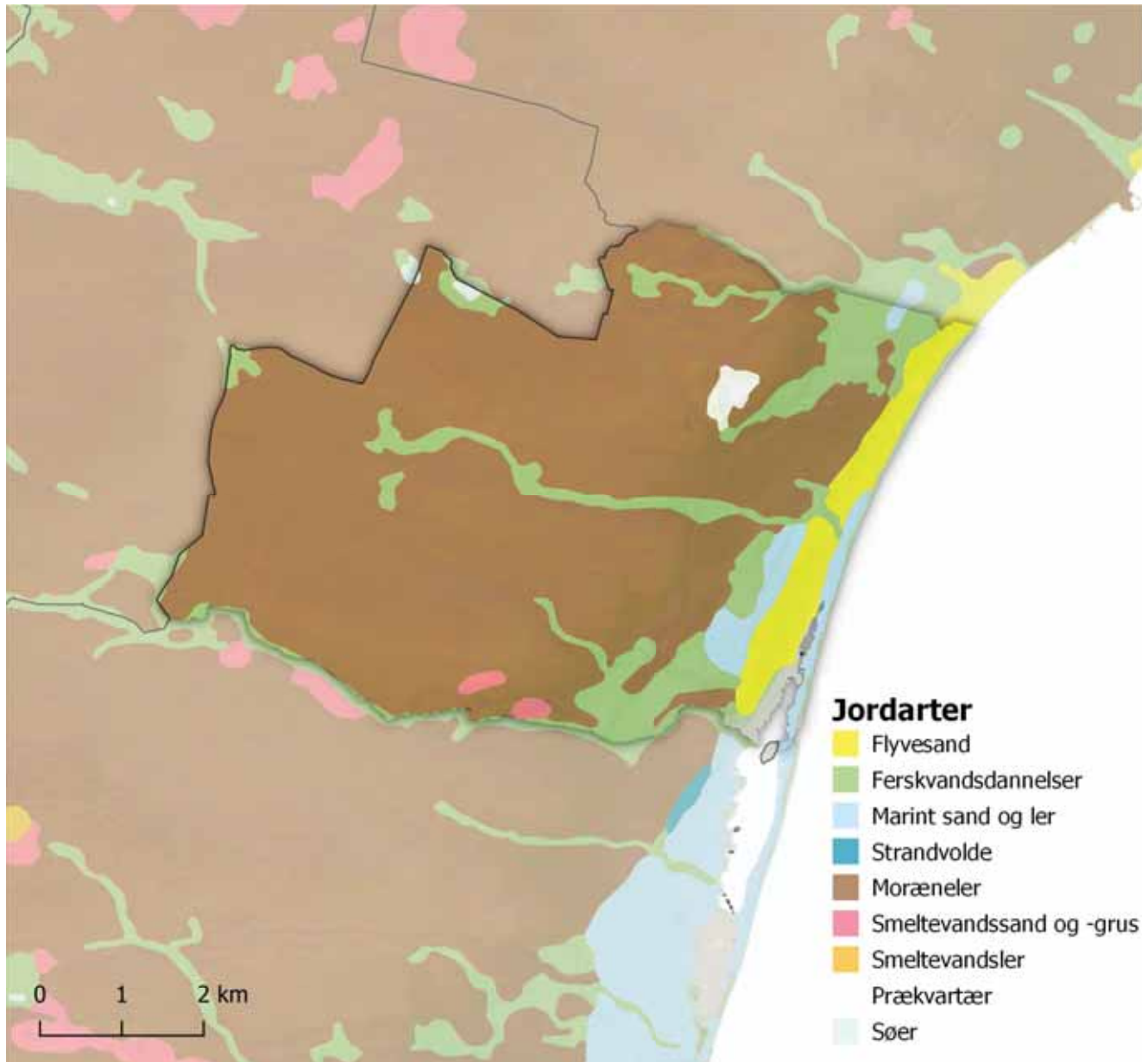
Figur 2.3: Jordartskort ©GEUS
